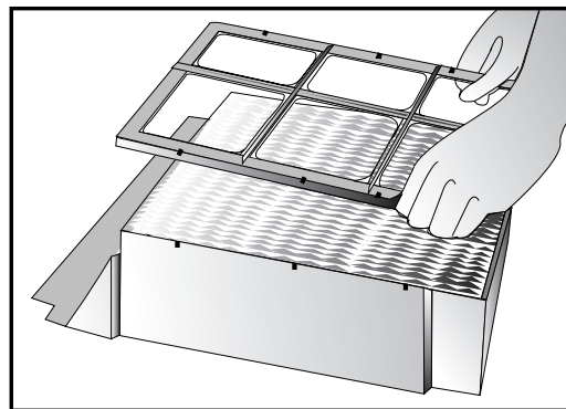
Démontage du châssis
