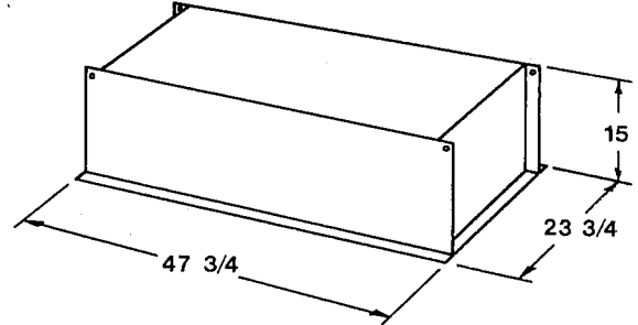
FIG. 2 - Dimensions approximatives d'installation en pouces.
