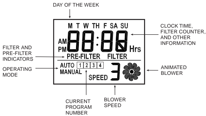
Fig. 5 - Alpha-numeric Display
