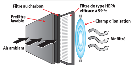
Fig. 1 Système de filtration en 4 étapes
