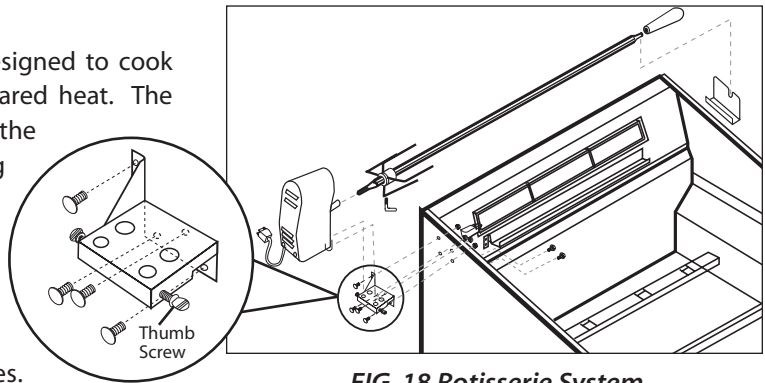
FIG. 18 Rotisserie System
