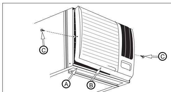
A Caisse C Panneau de façade décoratif B Vis de phillips
