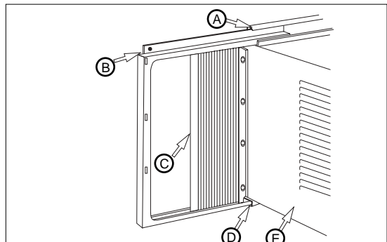
A Tringle supérieure C Bord de verrouillage B Cadre du panneau de remplissage D Tringle inférieure E Caisse
