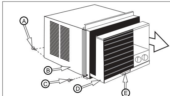
A Vis utilisées pour l'expédition D Châssis B Caisse E Poignée C Vis antivol
