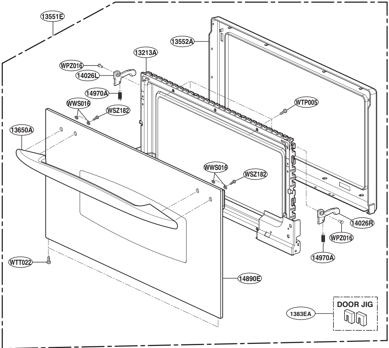
DOOR JIG
