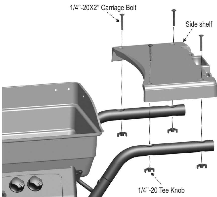
1/4"-20 Tee Knob Qty.8
