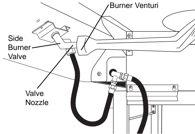
Orificios de la Mesa Lateral
