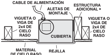
CUBIERTA MONTADA EN UNA VIGUETA DE 2x4 Se requiere una estructura adicional para las aletas de montaje. Descarga paralela a las viguetas.
