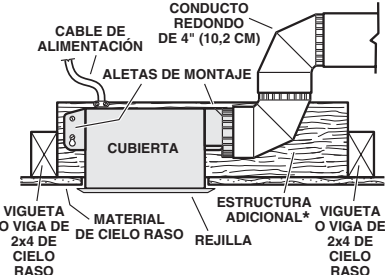
CUBIERTA MONTADA EN UNA VIGUETA DE 2x4 Se requiere una estructura adicional para las aletas de montaje. Descarga a 90° de las viguetas.
