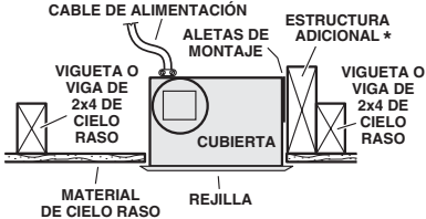
CUBIERTA MONTADA EN UNA VIGUETA DE 2x4 Se requiere una estructura adicional para las aletas de montaje. Descarga paralela a las viguetas.
