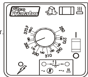
TERMOSTATO DE ESTADO SÓLIDO
