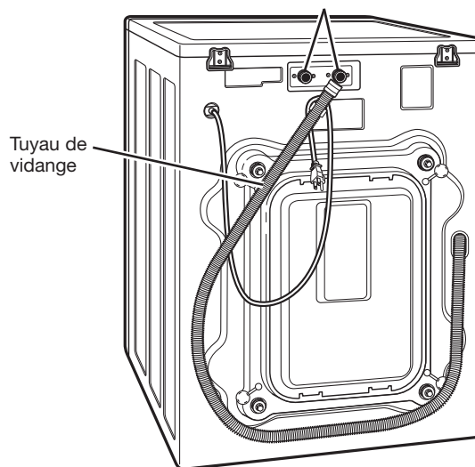
Arrière de la machine à laver
