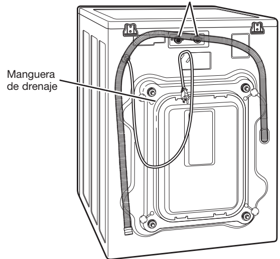
Parte trasera de la lavadora
