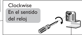
Chassis locking brackets Soportes que cierran el chasis
