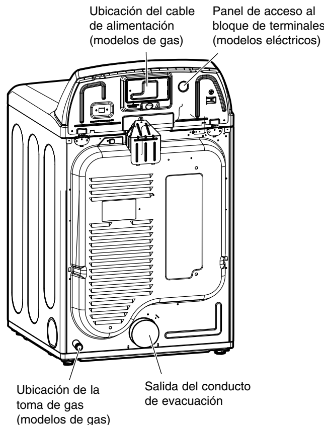
Parte posterior de la secadora
