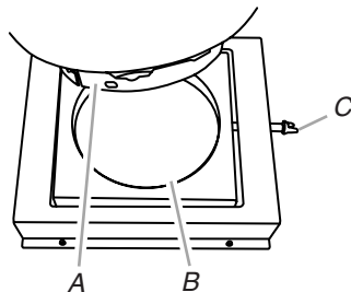
A. Collerette inférieure de la bouteille B. Trou de montage C. Vis de blocage
