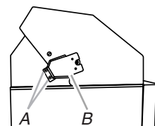
A. 2 screws B. Rotisserie bracket
