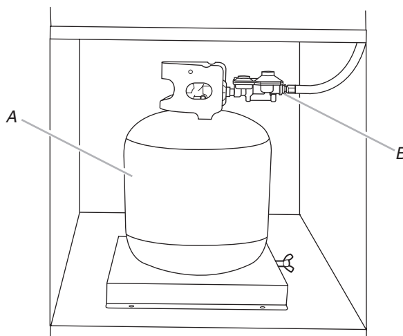
A. Bouteille de propane de 20 lb B. Ensemble détendeur/tuyau de raccordement
