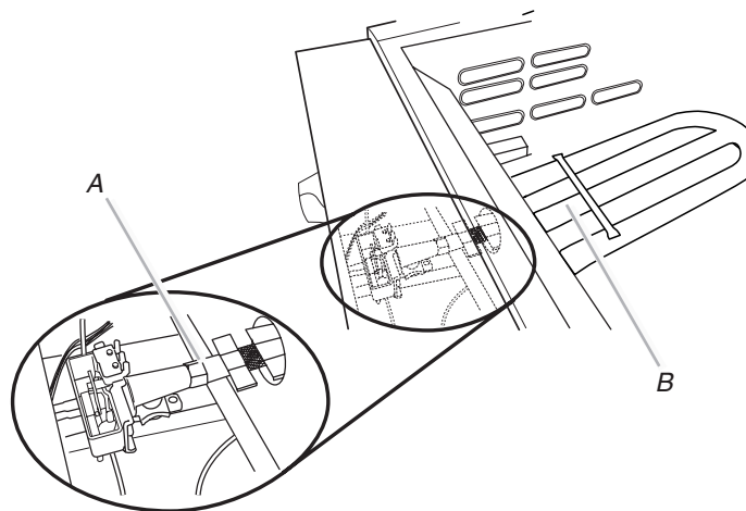
A. Raccordement du brûleur/de l'orifice B. Tube du milieu du brûleur
