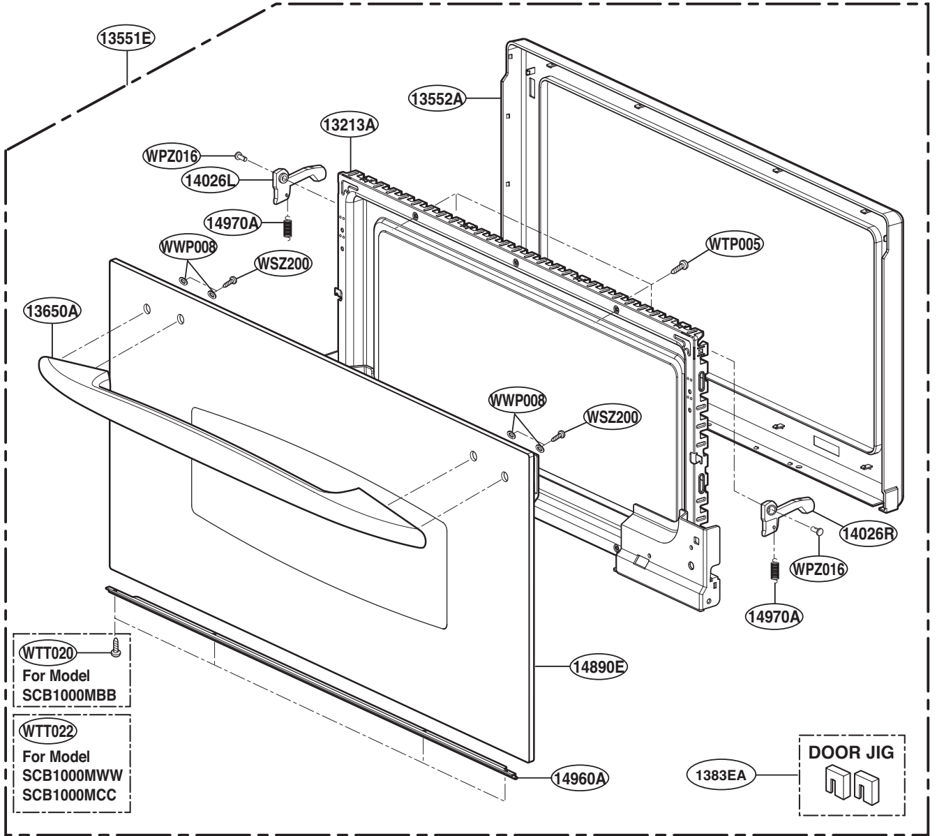
DOOR JIG
