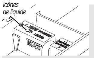
L'étiquette en avant pour détergent liquide
