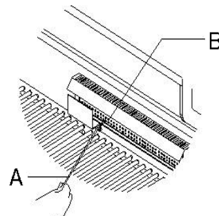
A. Extensión de encendido B. Quemador del rostizador
