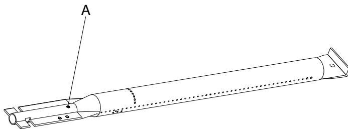
A. Vis de réglage de l'admission d'air
