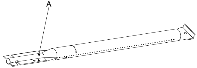
A. Tornillo de ajuste del obturador de aire
