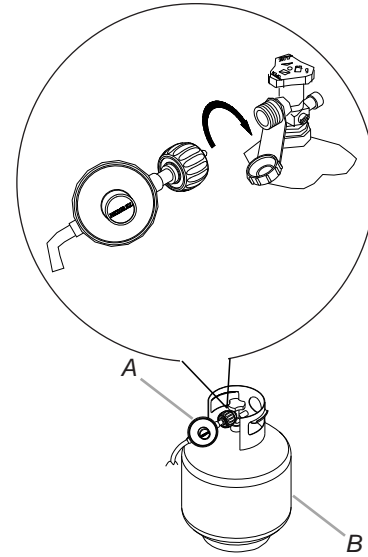
A. Bouteille de propane de 20 lb B. Ensemble détenteur/tuyau
