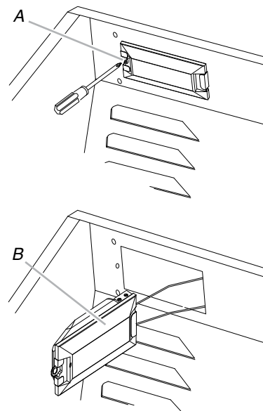
A. Vis B. Lampe
