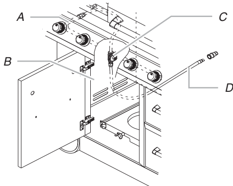
A. Distribuidor B. Panel lateral izquierdo C. Ensamblaje de regulador de presión/manguera de gas natural D. Manguera de gas en PVC de 10 pies (3,0 m)
