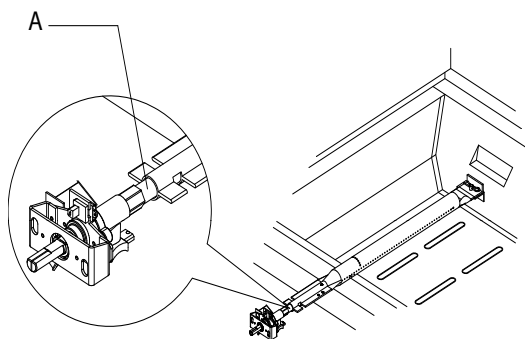
A. Raccordement brûleur/gicleur
