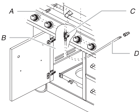
A. Tubulure de distribution B. Panneau de gauche C. Ensemble détendeur pour gaz naturel/tuyau D. Tuyau gris
