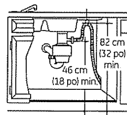
Installation avec broyeur à déchets
