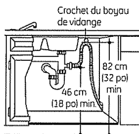
Installation avec raccord en T
