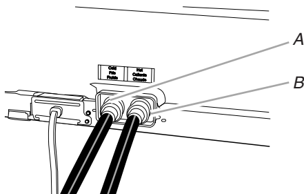
A. Electrovanne d'alimentation - bleu = eau froide B. Electrovanne d'alimentation - rouge = eau chaude
