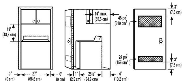
A. Vue avant B. Vue de profil C. Porte de placard avec ouvertures d'aération
