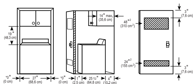
1. Vue avant 2. Vue de profil 3. Porte de placard avec ouvertures d'aération
