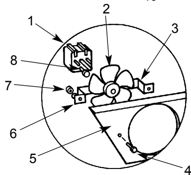
Evaporator Fan
