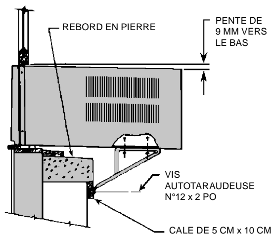
Figure 3A PLAN DE MONTAGE TYPIQUE
