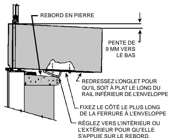
Figure 4A PLAN DE FERRURE DE SUPPORT INVERSÉ
