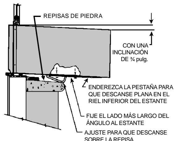
Figura 4A ESQUEMA DE ÁNGULOS DE SOPORTE INVERTIDOS
