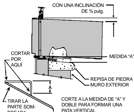
Figura 2A ESQUEMA DE UNA INSTALACIÓN MODIFICADA
