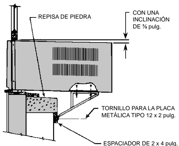
Figura 3A ESQUEMA DE UNA INSTALACIÓN TÍPICA
