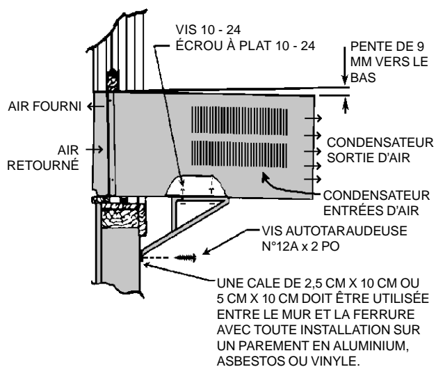
Figure 1A Figure 1A PLAN DE MONTAGE TYPIQUE
