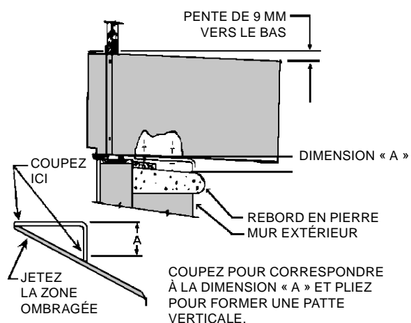
Figure 2A PLAN DE MONTAGE MODIFIÉ
