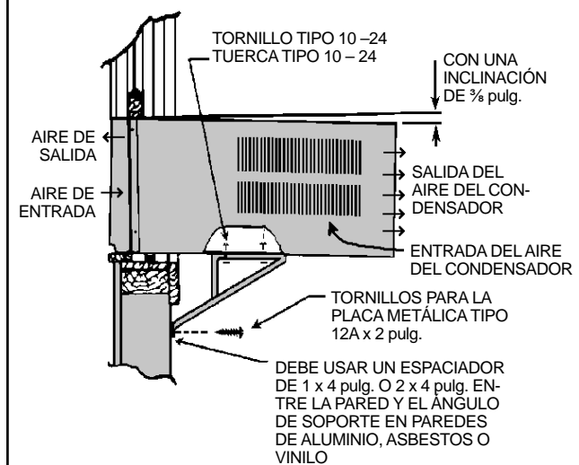
Figura 1A ESQUEMA DE UNA INSTALACIÓN TÍPICA
