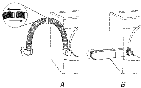
A. Installation au-dessus de la sècheuse (aussi disponible avec un coude décalé)
