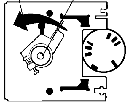
Vue avant de la minuterie
