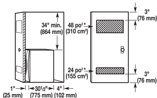
A. Vue latérale - placard ou endroit exigu B. Porte de placard avec oriïces d'entrée d'air
