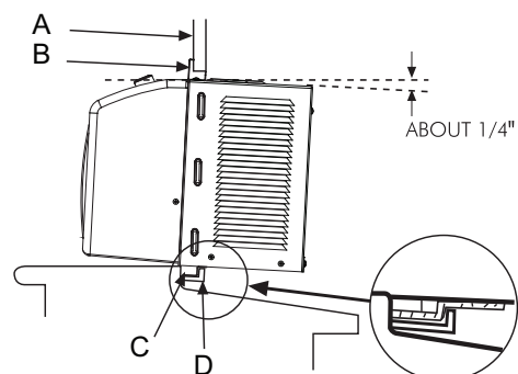
A. Cadre de la fenêtre B. Guide supérieur C. Guide inférieur D. Console d'angle du fond
