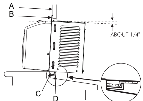
A. VENTANA B. GUÍA SUP C. GUÍA D. ÁNGULO
