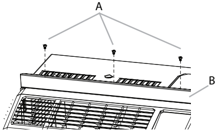
A. Vis de \frac{13}{32} " B. Glissière supérieure
