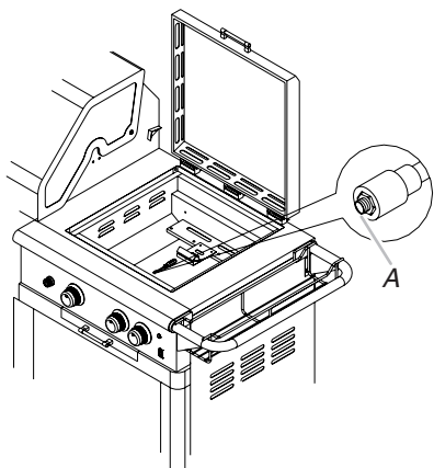
A. Orificio
