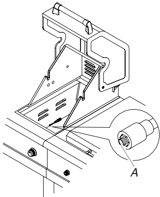
A. Gicleur
