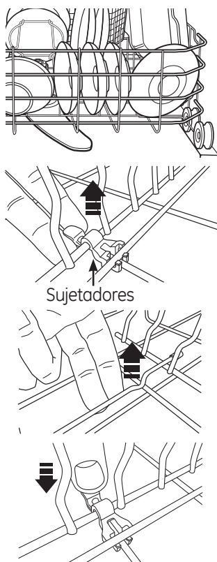
Estante inférieur-Configuraciones de 8 lugares - GDF510, GDF520 & ADT521
