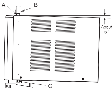
A. Guide supérieur B. Guillotine de fenêtre C. Guide inférieur
