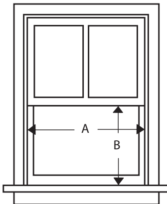
A. 28\frac{3}{8} " (72.1 cm) como mínimo B. 17\frac{3}{8} " (44.1 cm) como mínimo
