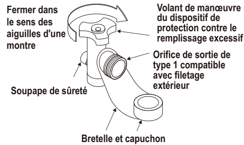
N'utilisez pas de bouchon de transport de produits pétroliers (pièce en plastique avec filetage extérieur)! Il empêchera le dispositif de sûreté de la valve de fonctionner.
