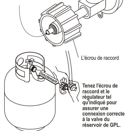
Le mamelon doit être centré dans la valve du réservoir de GPL.
