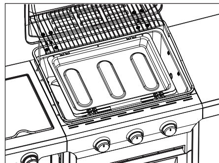
Colocación correcta de la bandeja de carbón
