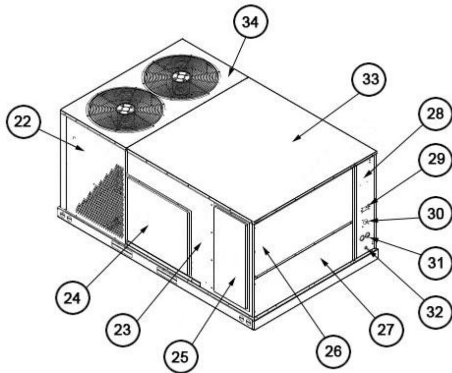
Exterior - Back 072-151
