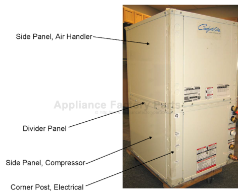
HRV Sheetmetal Parts
