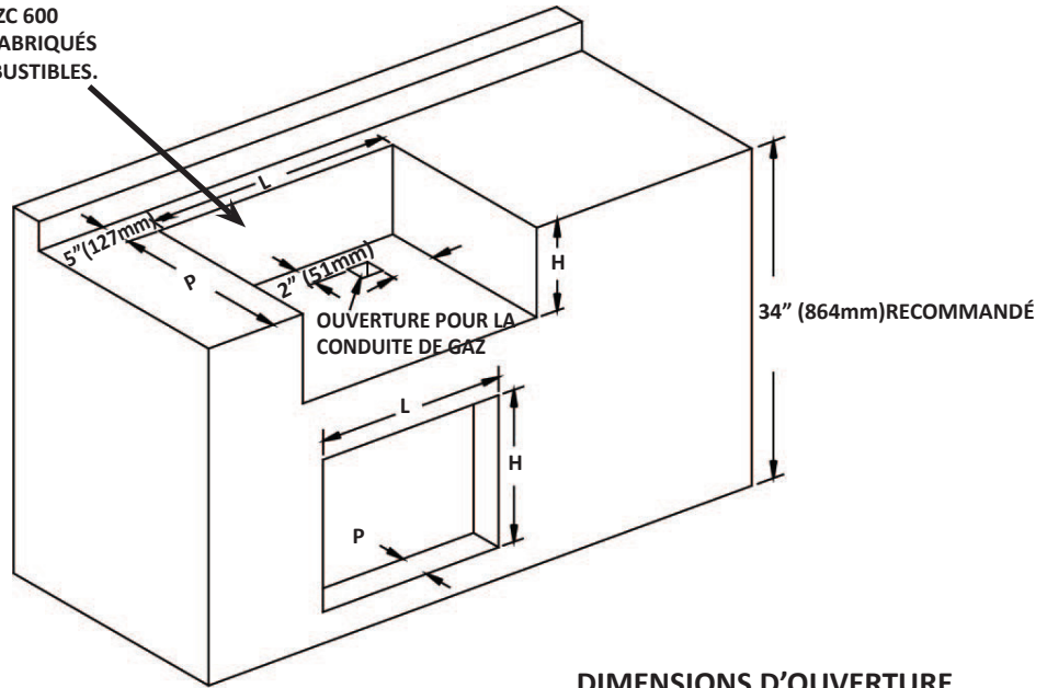
DIMENSIONS D'OUVERTURE
