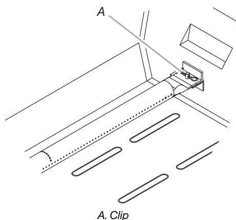
A. Clip
