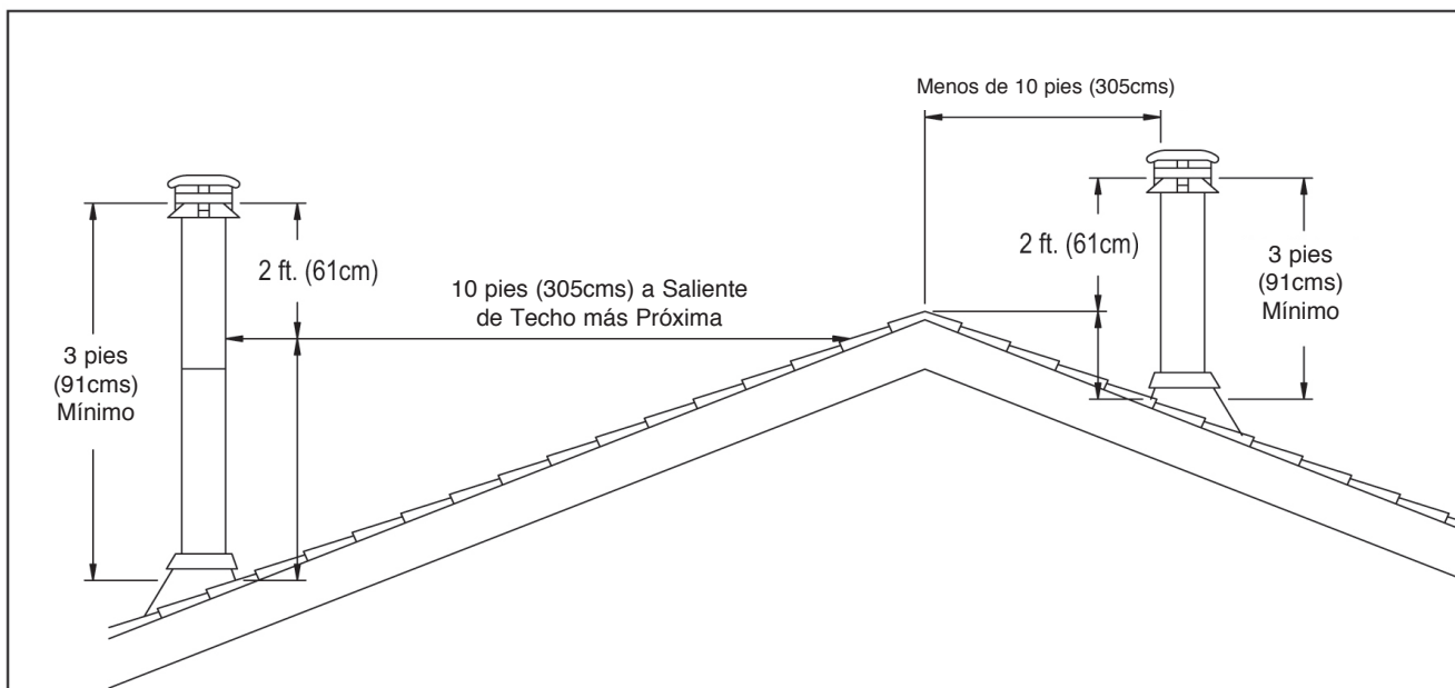
Techo Inclinado
