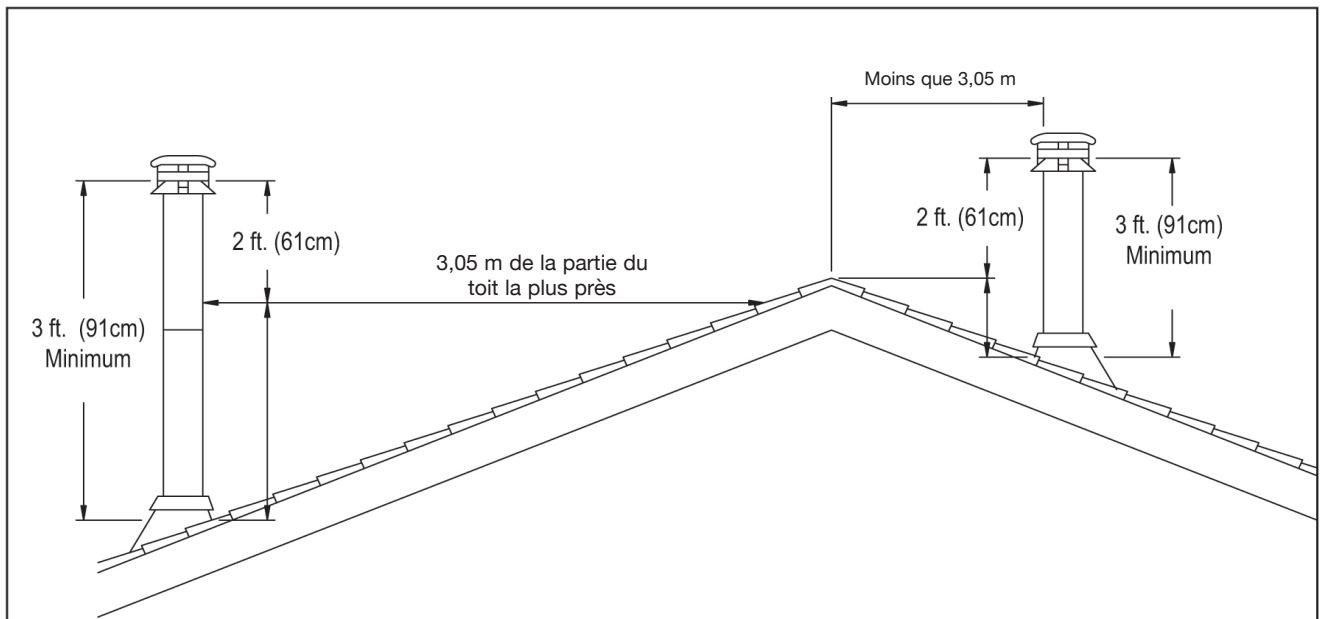
Toit incliné
