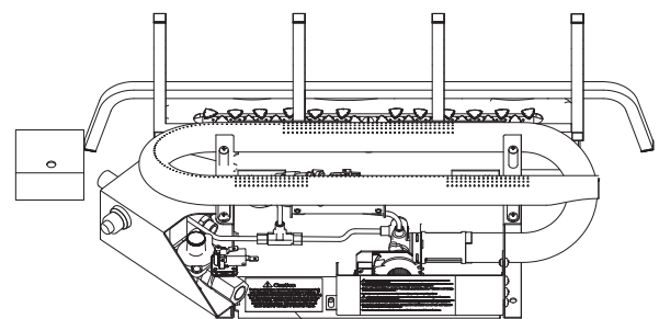
Fig. 38 - Ubicación de la etiqueta de precaución (vista de la parte trasera de la unidad)
