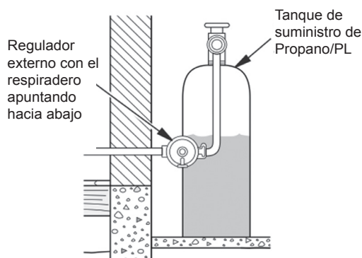
Fig. 13 - Conversión del regulador
