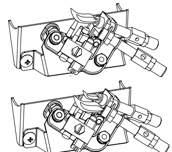
Fig. 16 - Piloto
