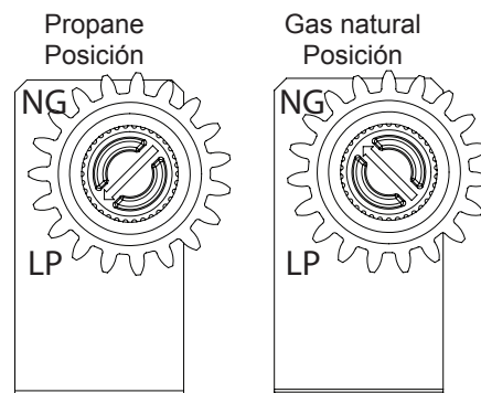
Fig. 8 - Válvula selectora
