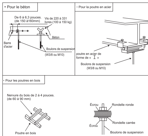
Fig. 3.2.1 Fixation des boulons de suspension
