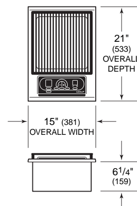
Model IG15/S
