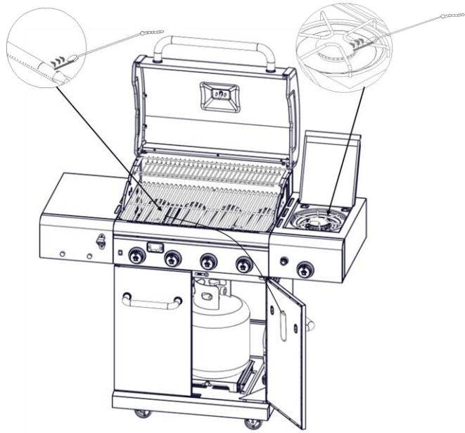
Quemador principal
