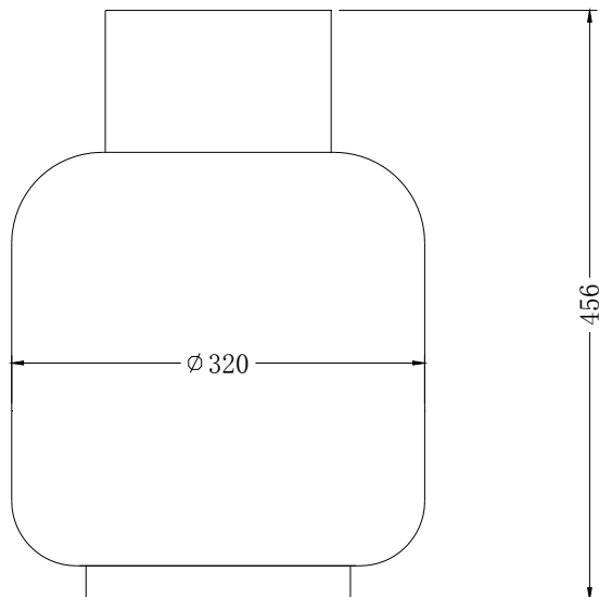
Réservoir de propane: hauteur = 456mm, diamètre = 320mm
