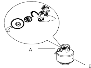
A. Ensemble détendeur/tuyau d'alimentation B. Bouteille de propane (20 lb)
