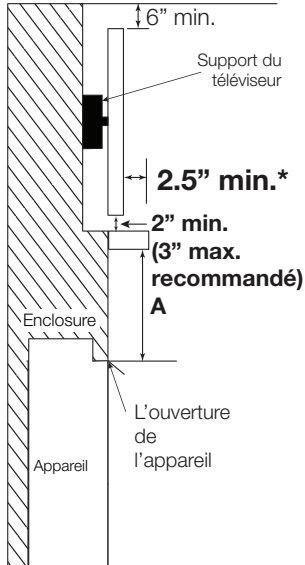
Installation partiellement enchâssées avec un manteau
