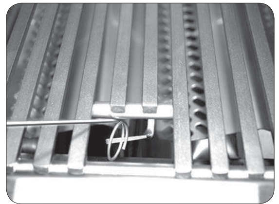
Fig. 28-2 - Éclairage manuel
